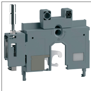
mechanisches Verriegelungset für 3P und 4P P160 (Bowdenzug)
