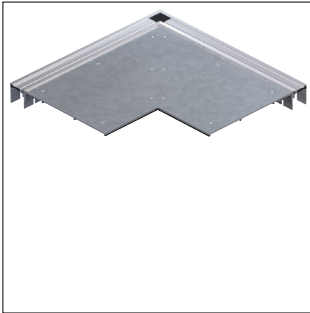
Angle plat Covercle à rebords Intérieur pour Canal de sol BKB 300x80
