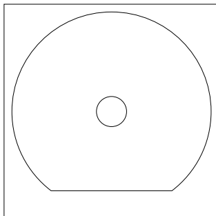
Kunstst.unterl. f. Glasendplatte f. Drehschalter-/Taster Serie Glas klar (1094)
