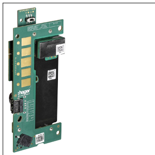
Carte d'interface HMI pour EVCS witty plus/pro
