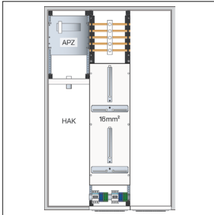
Zähleranschlussssäule 131, universZ, 2ZP, 3.HZ, 5-polig, Basis, Vorb. f. 4ZP, APZ
